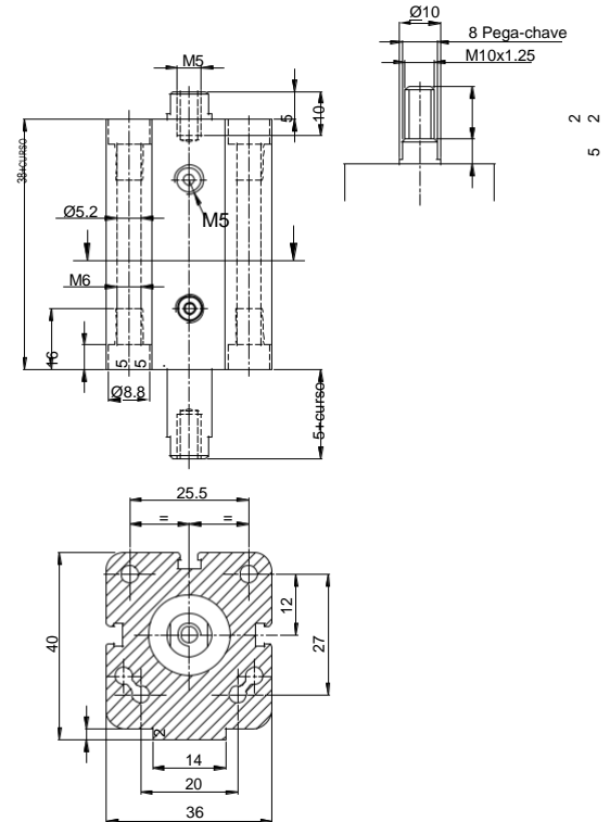
Cilindro com Haste Passante Ø 32
