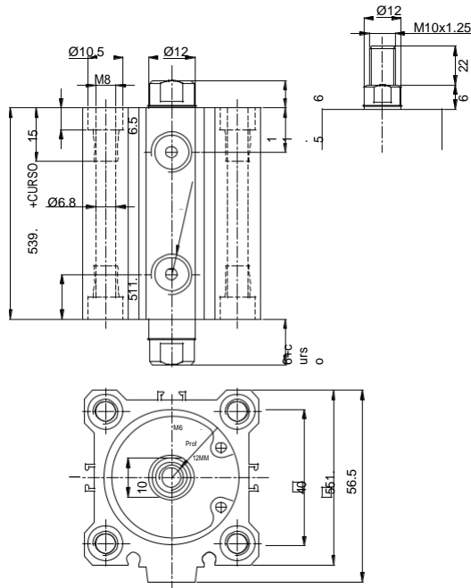
Cilindro com Haste Passante Ø 40
