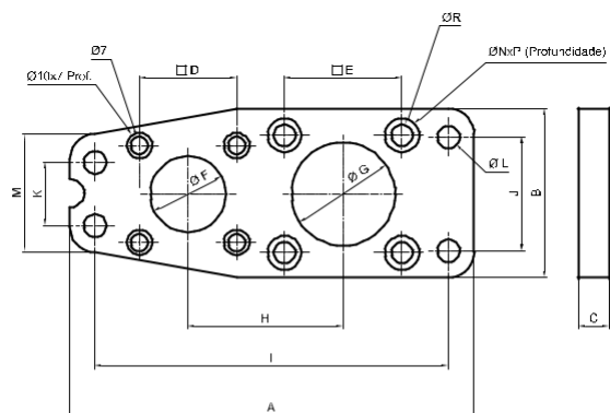
Diâmetro 100
