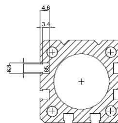
Tubo Europa com canal para sensor.
