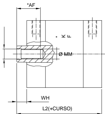
Haste com Rosca Fêmea
