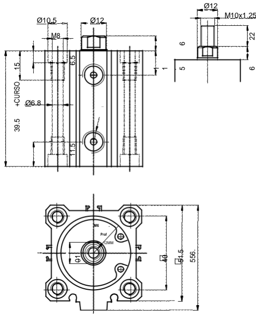
Cilindro Ø 40
