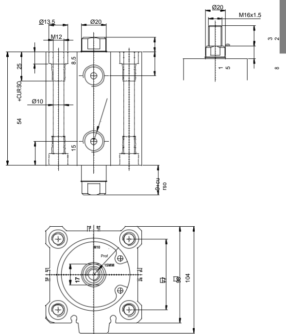
Cilindro com Haste Passante Ø 80
