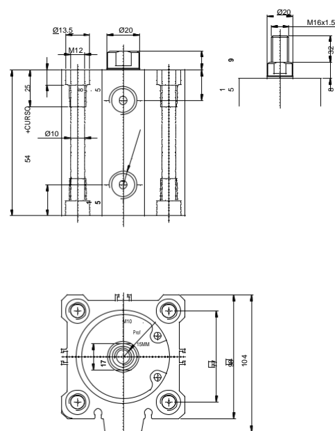
Cilindro Ø 80
