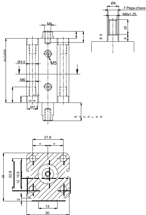
Cilindro com Haste Passante Ø 16
