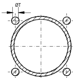
Tubo para cilindros tirantados.
