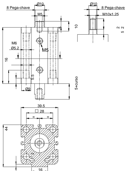
Cilindro com Haste Passante Ø 25
