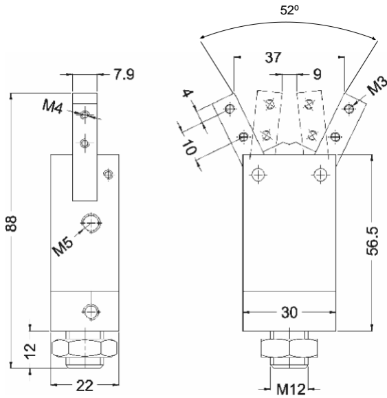
Garra Ø16
