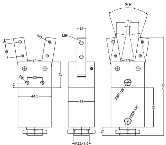
Garra Ø32
