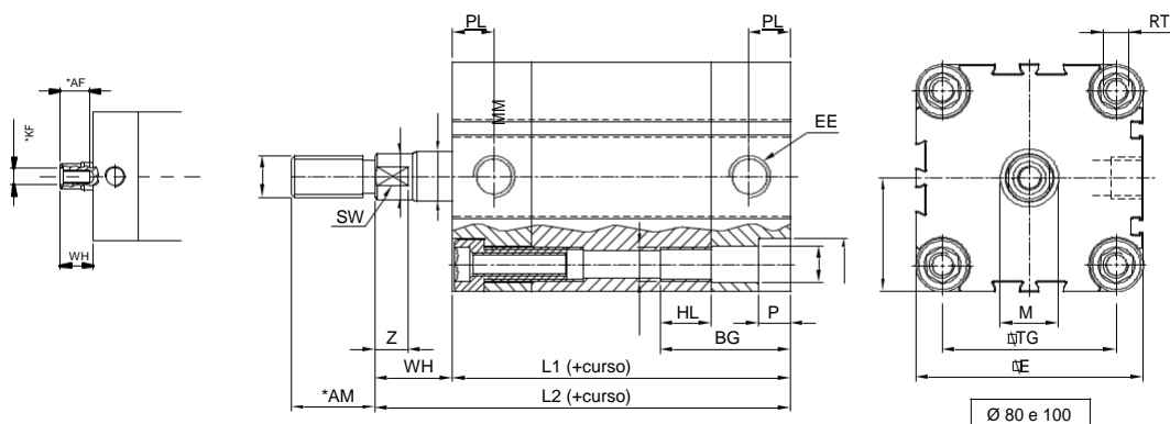
Ø 80 e 100
