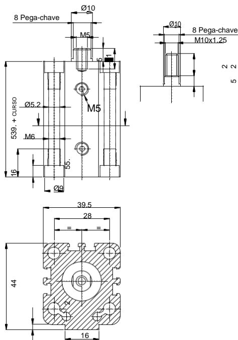
Cilindro Ø 25
