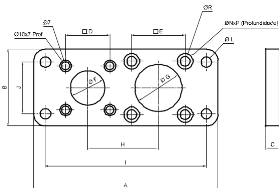
Diâmetro 32-80
