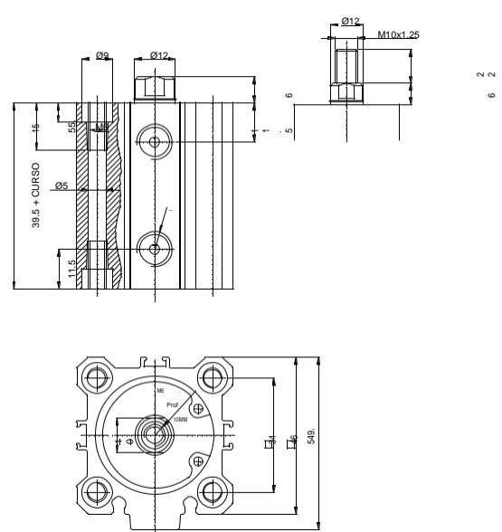
Cilindro Ø 32
