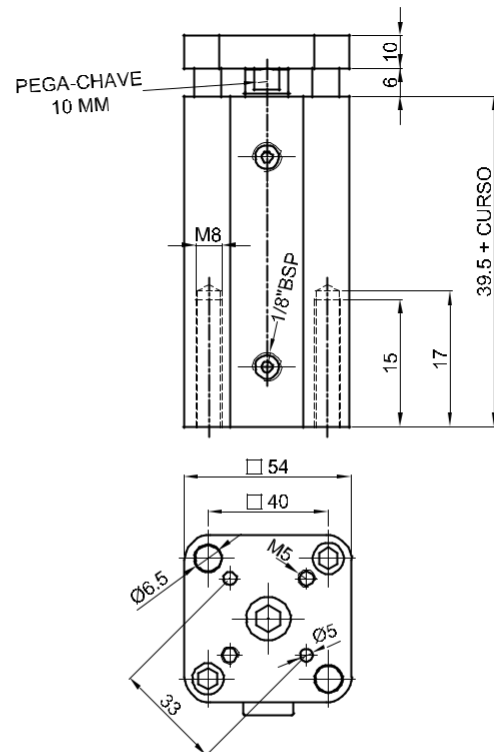
Cilindro com Antigo Ø 40
