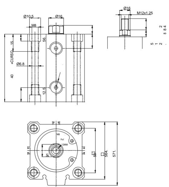
Cilindro Ø 50
