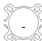
PERFILADO ISO Ø32 AO Ø100
