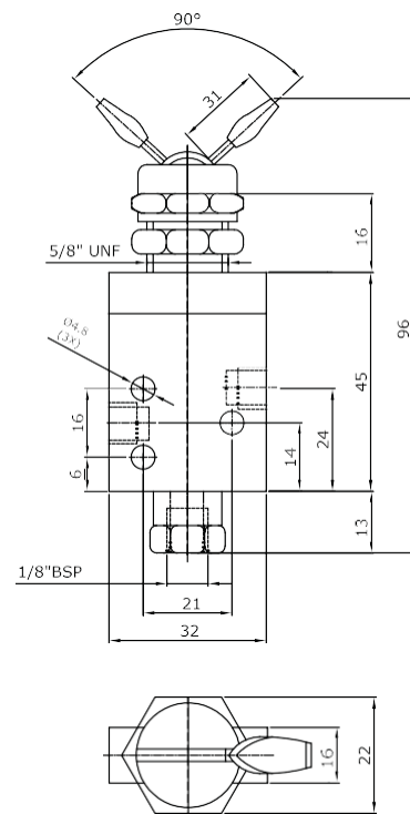
Válvula Alavanca/Trava - Referência: 3311
