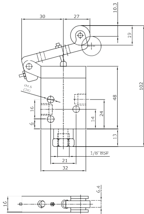
Válvula Rolete/Mola - Referência: 3370
