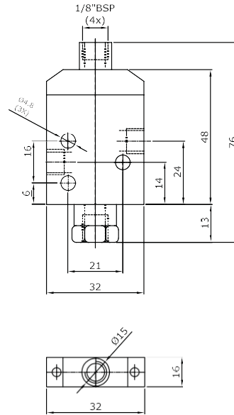
Válvula Pino/Mola - Referência: 3360
